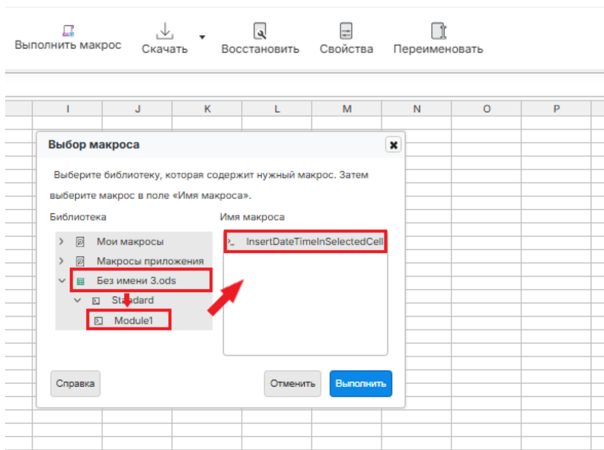
Рисунок 53. Поиск макроса в библиотеке
