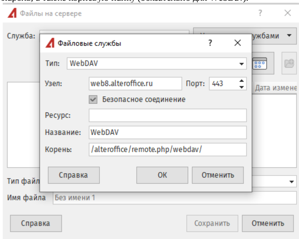
Рис. 27. Настройка файловых служб
