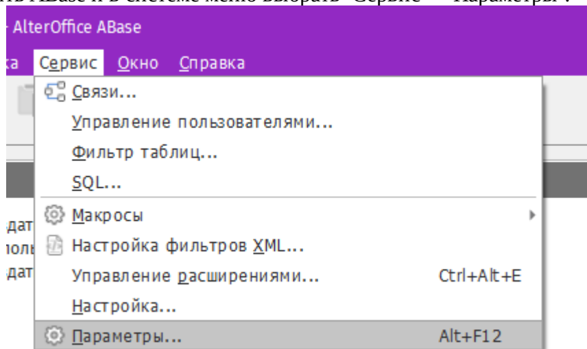
Рис. 24. Настройка JRE
