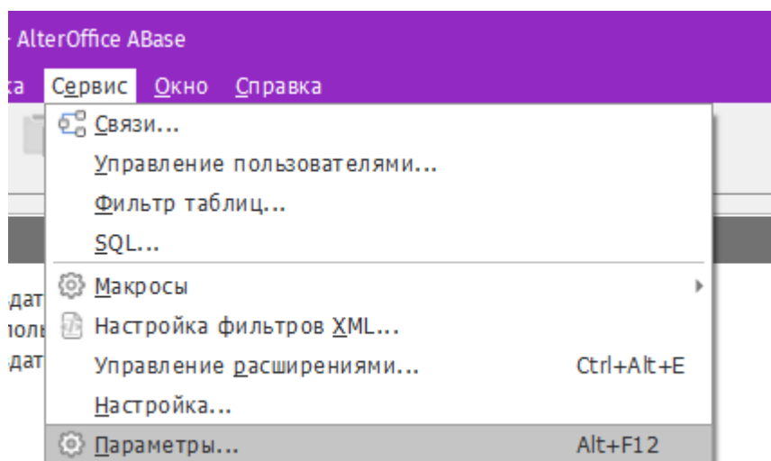
Рис. 18. Настройка JRE
